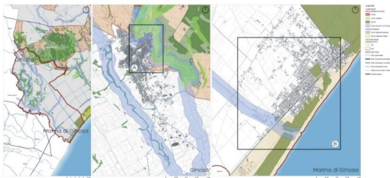
Ginosa - Landslide risk
