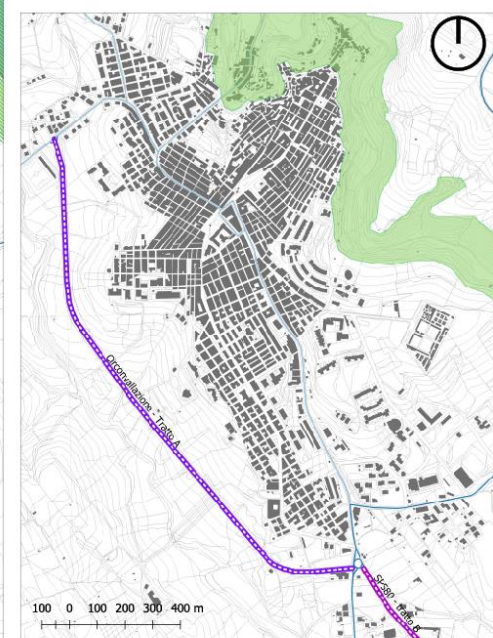
DETTAGLIO PISTE CICLABILI URBANE E PERIURBANE ESISTENTI E DA RIQUALIFICARE
