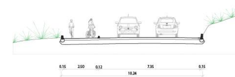
SEZIONE TIPO - TRATTO A
