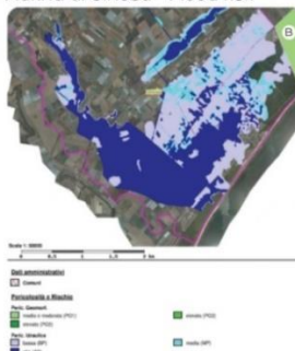
Marina di Ginosa - Flood risk
