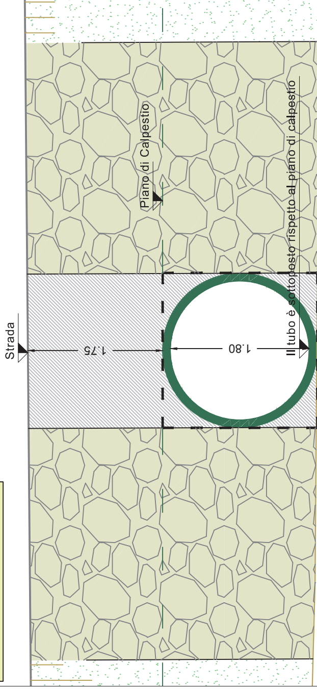
Sezione del Tombino Circonvallazione 4
