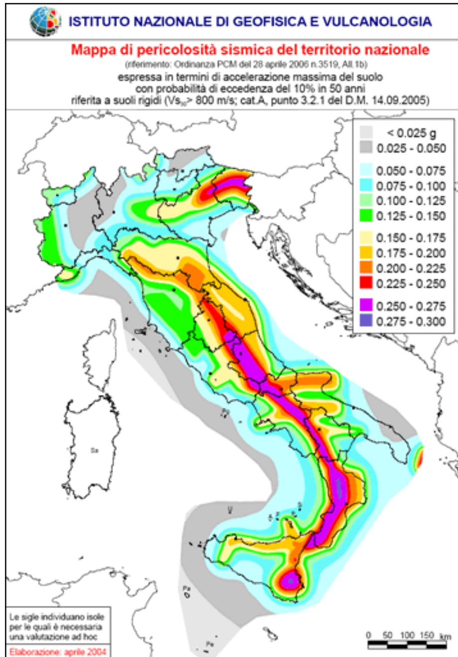
Fig. 6: Mappa di pericolosità sismica del territorio
