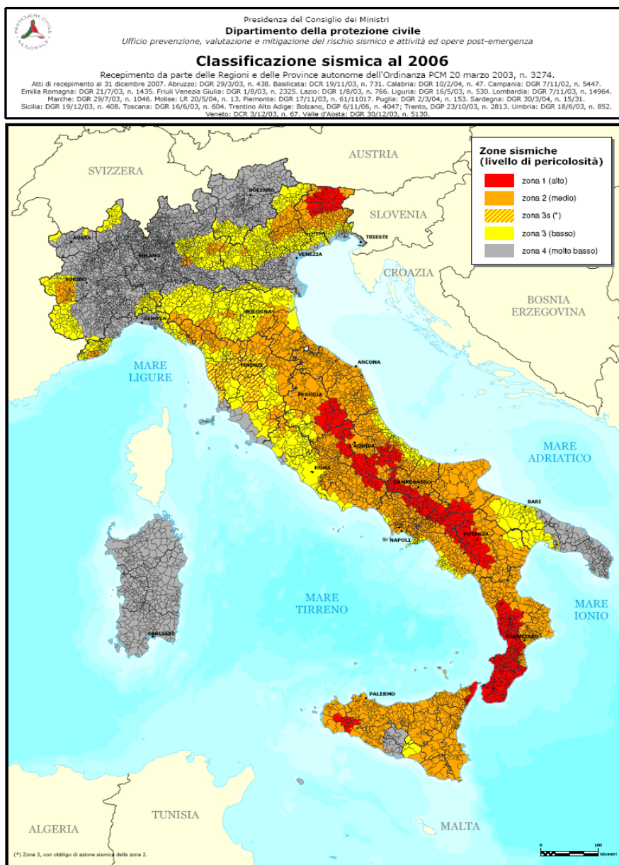
Fig. 5: Zone sismiche al 2006
