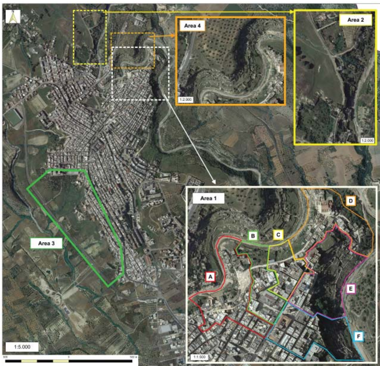
Fig.47: Zone di intervento: 1) Centro storico; 2) Via Pescarella; 3) Versante T. Gravinella; 4) Sinistra T. Lagnone
