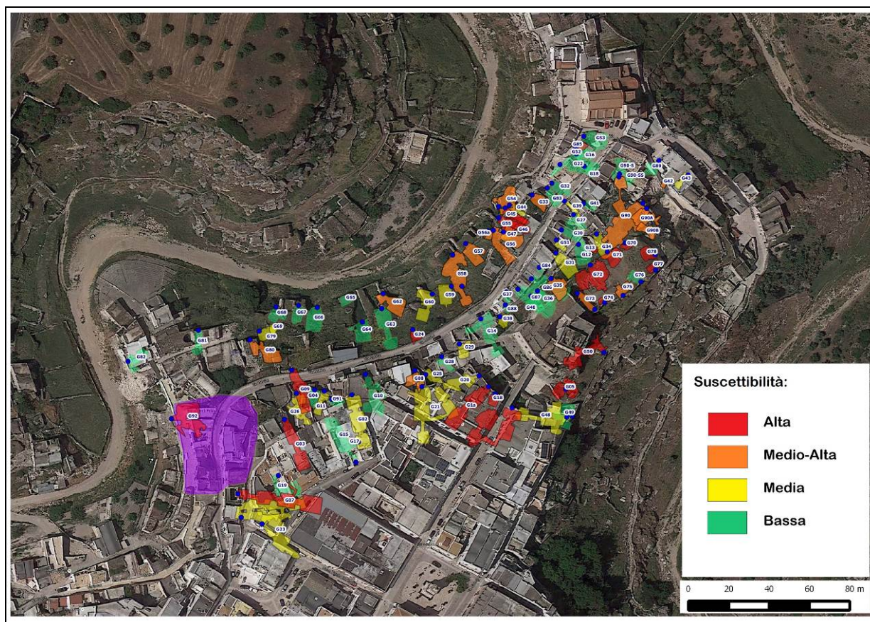
Fig. 35: Suscettibilità al crollo delle cavità rilevate - CNR-IRPI
