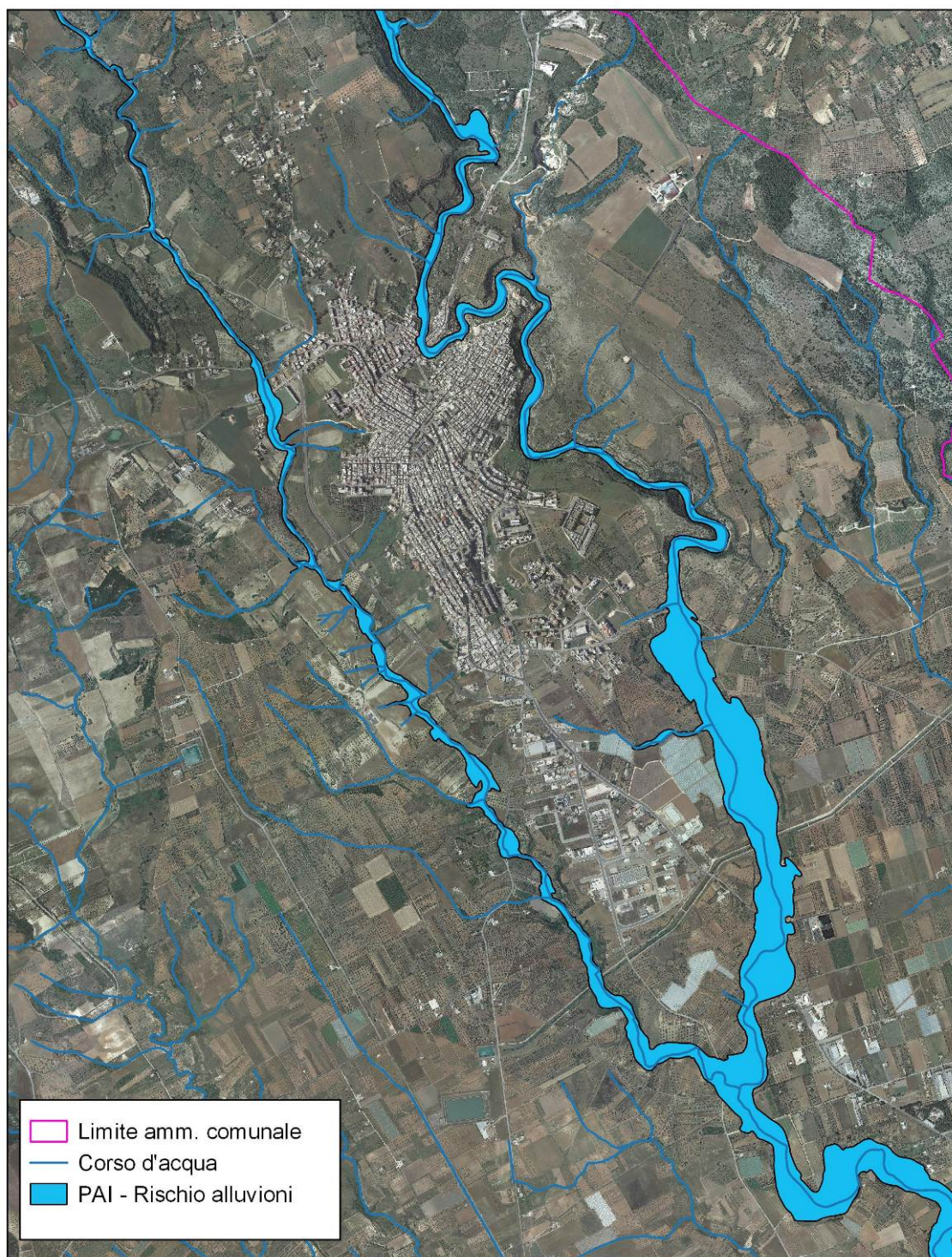
Fig. 11: Ginosa, rischio alluvioni (AdB Basilicata – PAI)
