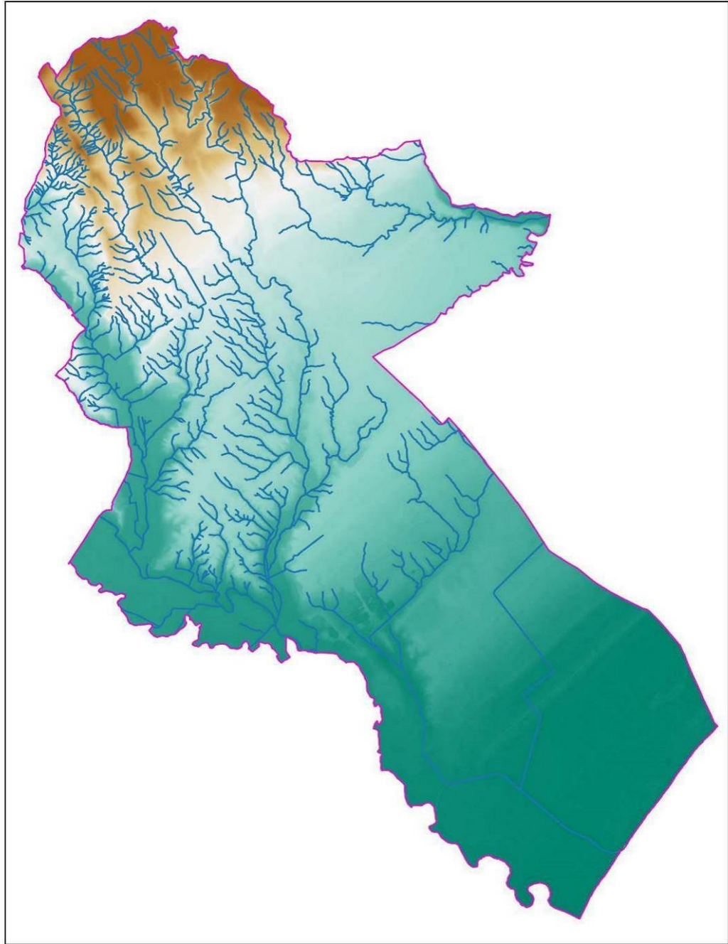
Fig. 1: DTM - Modello digitale del terreno
