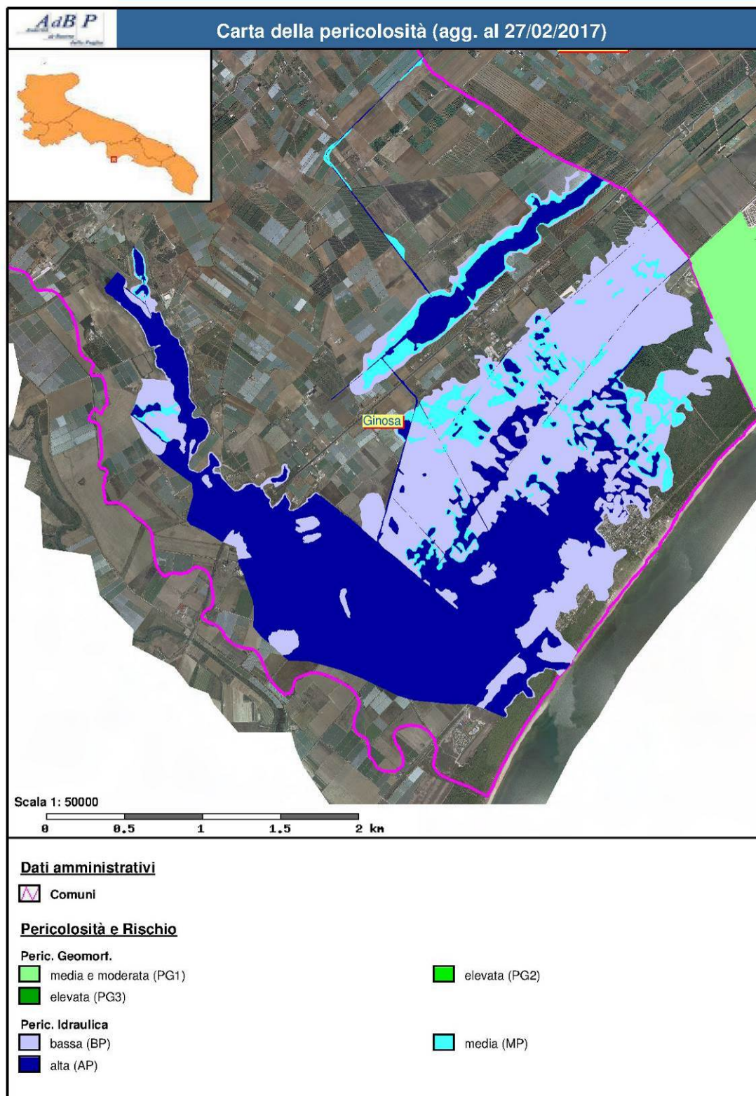
Fig. 12: Marina di Ginosa, rischio alluvioni (AdB Puglia – PAI)
