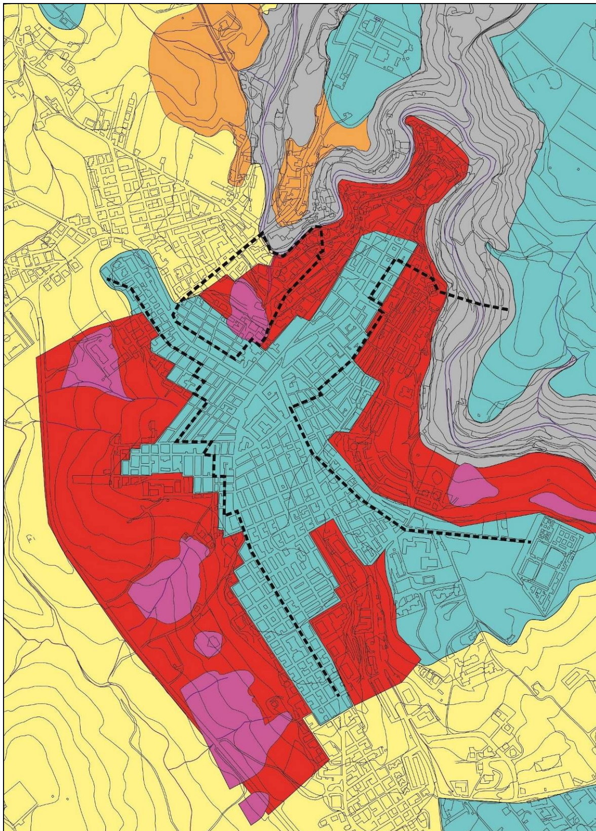
Fig. 37: Zonizzazione e suscettività d'uso del territorio (PRG - 1997)
