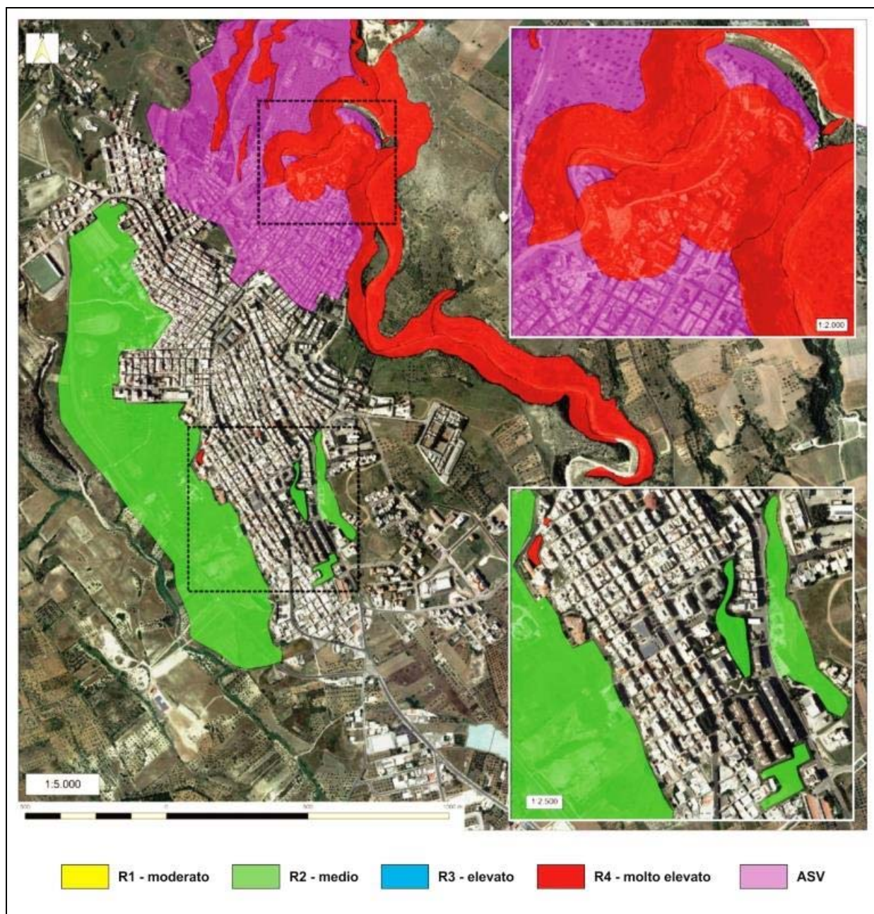
Fig. 46: Proposta di nuova perimetrazione delle aree a rischio geomorfologico (Tav. B4)
