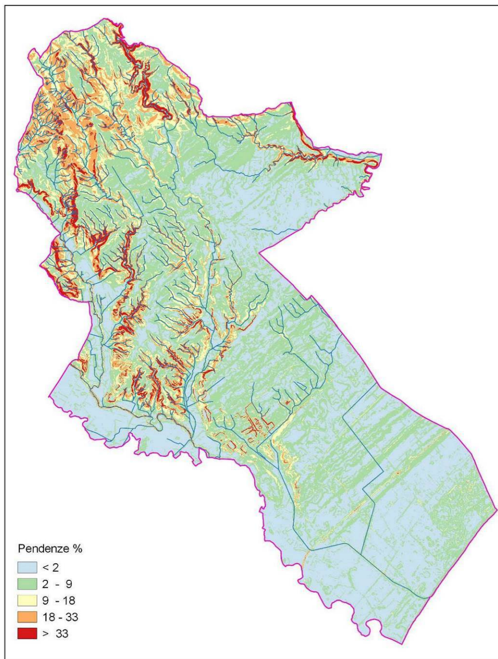
Fig. 3: Carta dell'acclività del terreno
