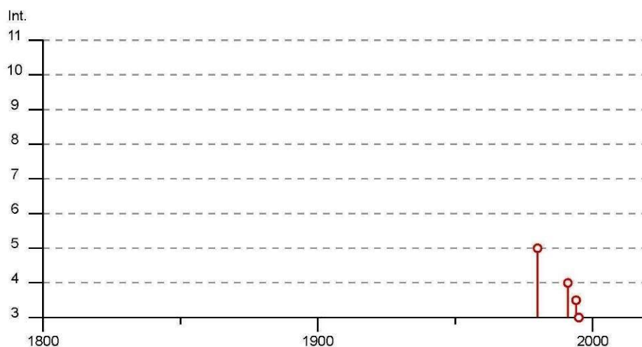
Fig. 9: Storia sismica di Marina di Ginosa, DBMI15 (2016)
