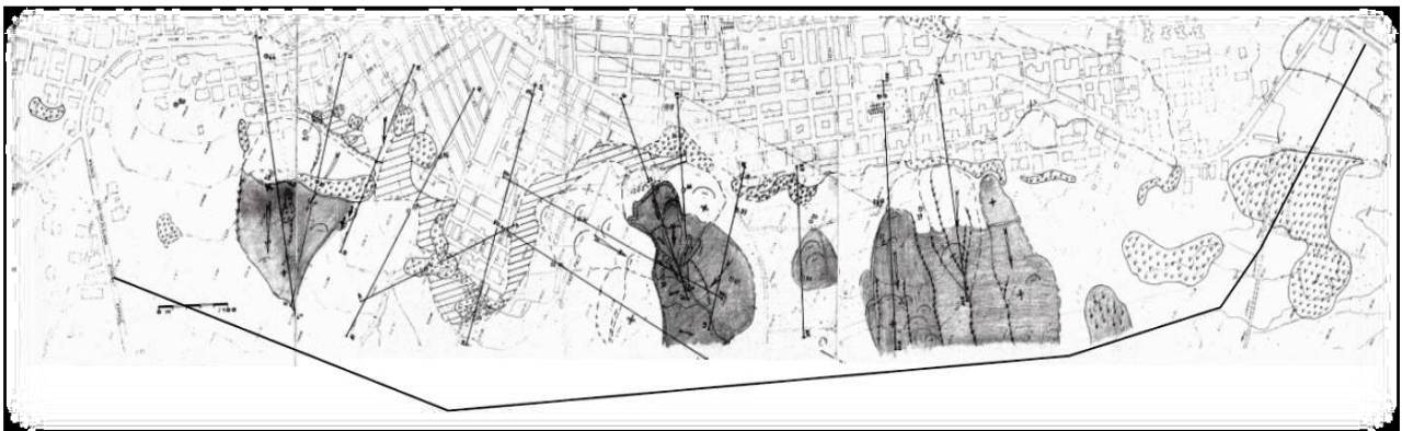
Fig. 39: Gruppi di antiche frane lungo il pendio prospiciente il T. Gravinella (Melidoro, 1985)
