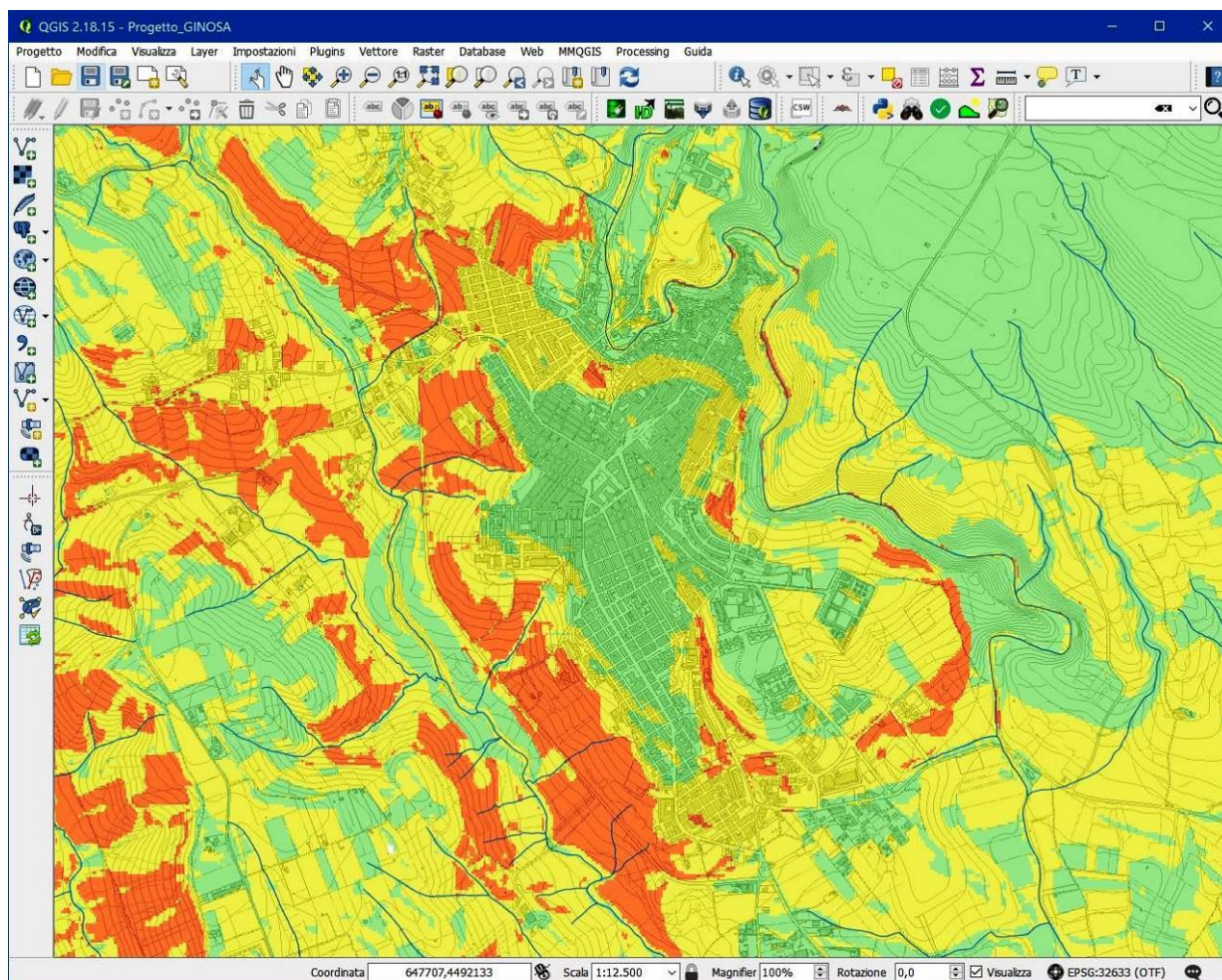
Fig. 41: Instabilità potenziale del versante
