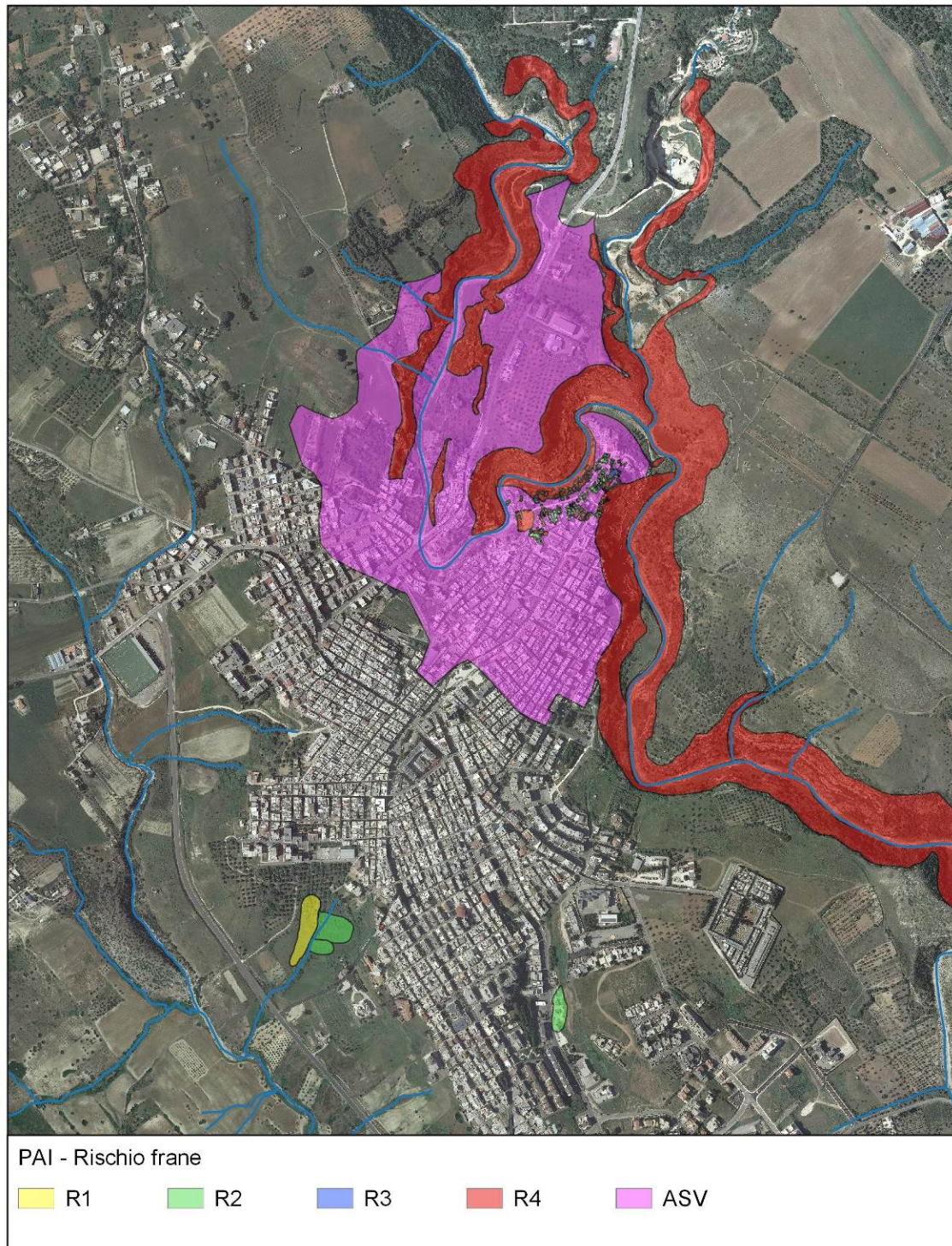
Fig. 10: Ginosa, rischio frane (AdB Basilicata – PAI)
