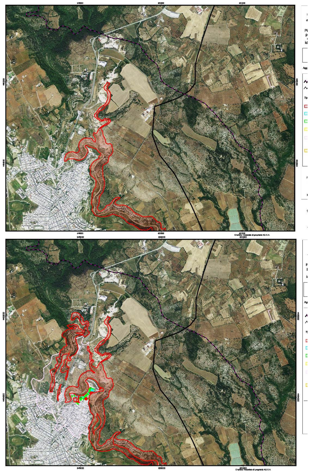
Fig. 42: PAI AdB Basilicata, agg. 2013 (in alto), agg. 2015 (in basso)
