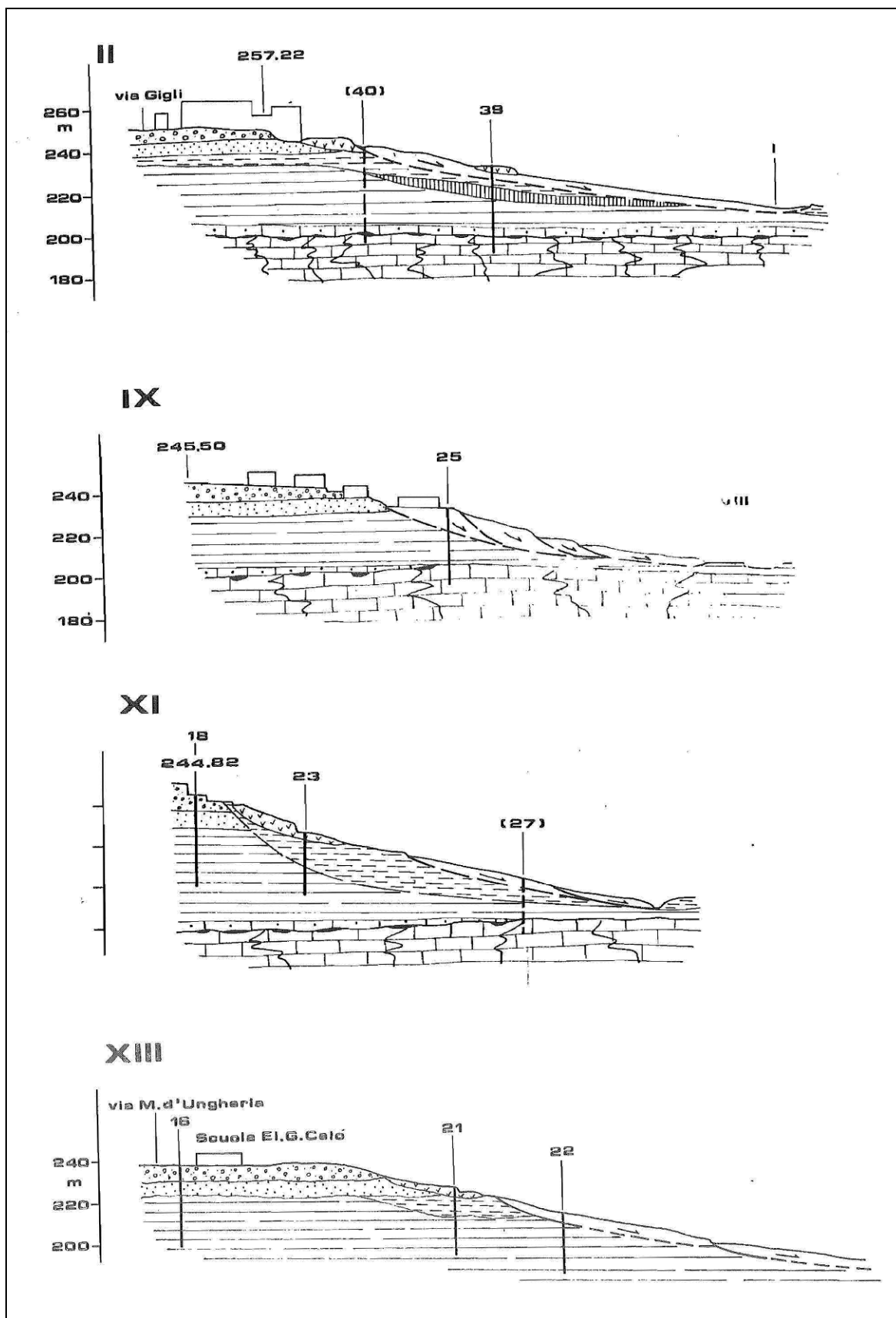
Fig. 40: Sezioni geologiche (Melidoro, 1985)
