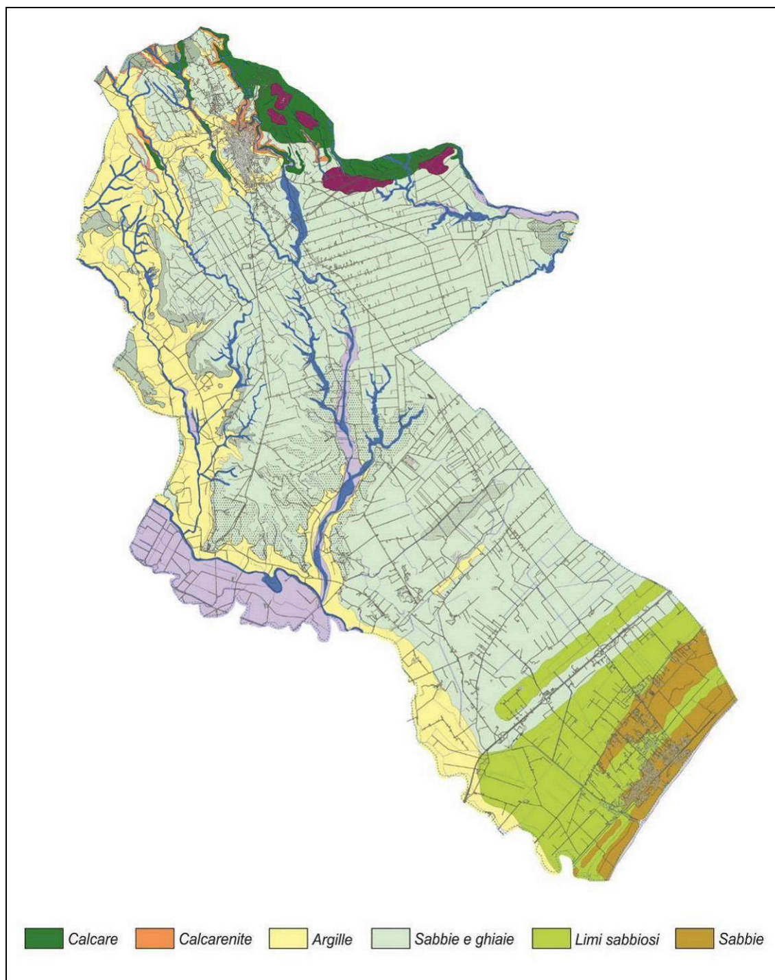
Fig. 1: Carta geolitologica del territorio di Ginosa
