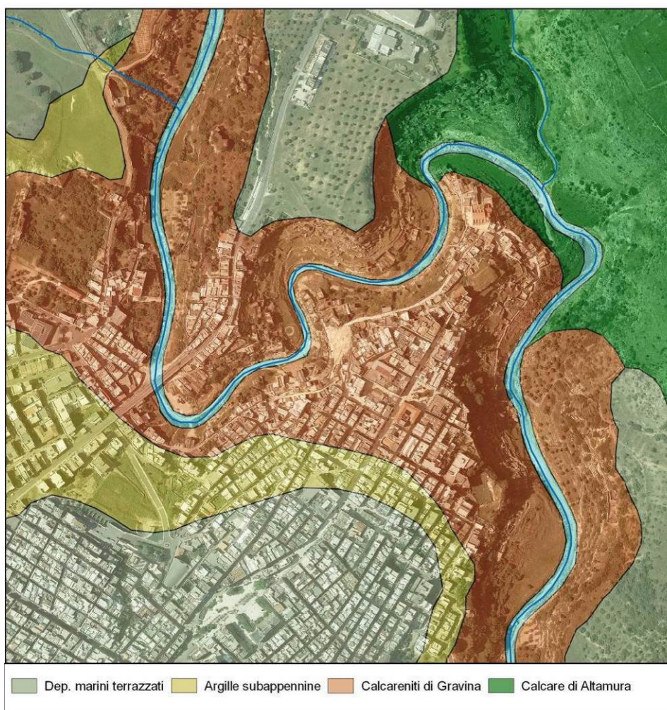
Fig. 14: Ginosa, centro storico: stralcio carta geologica
