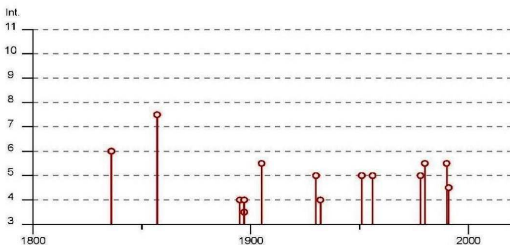
Fig. 8: Storia sismica di Ginosa, DBMI15 (2016)
