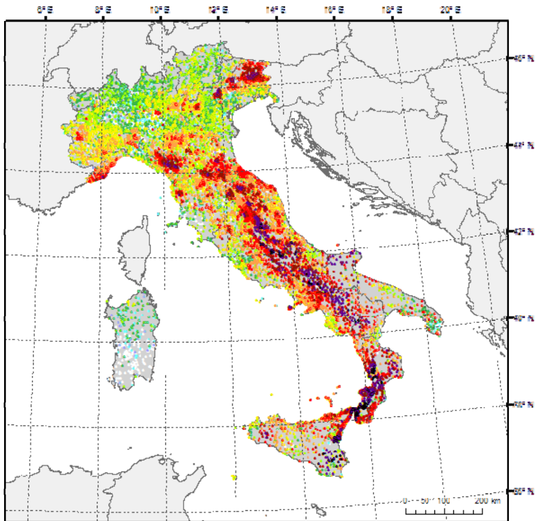
Fig. 7: Distribuzione delle intensità massime osservate per le 15213 località italiane
